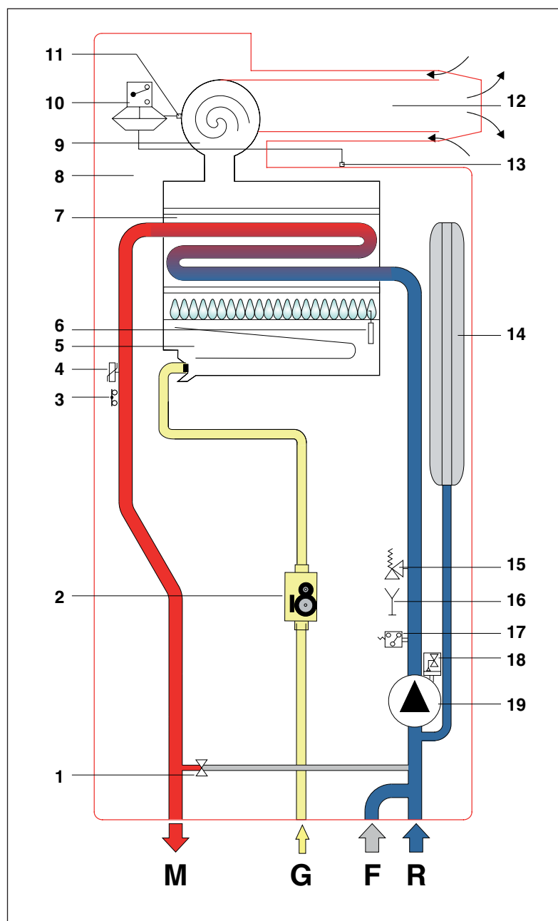
Рис. 7 Гидравлические схемы - RTFS
