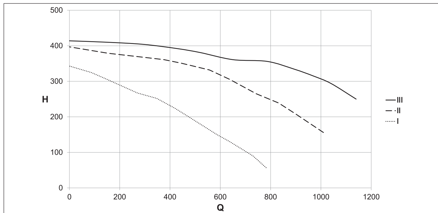
Рис. 17 Располагаемый напор CTFS 24
