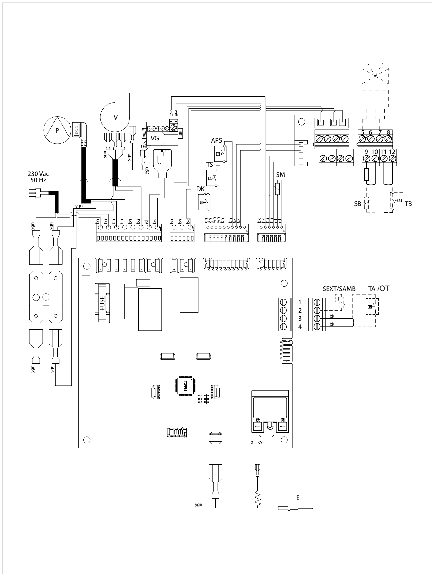
Рис. 21 Электрическая схема RTFS
