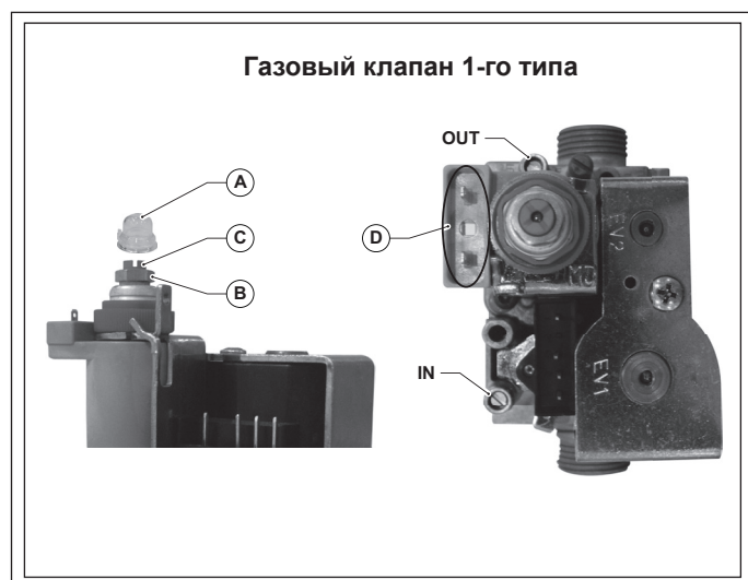
Рис. 27 Газовый клапан 1-го типа - 2-го типа
