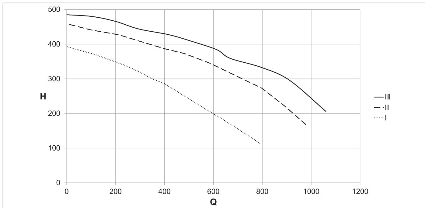
Рис. 18 Располагаемый напор CTFS 28
