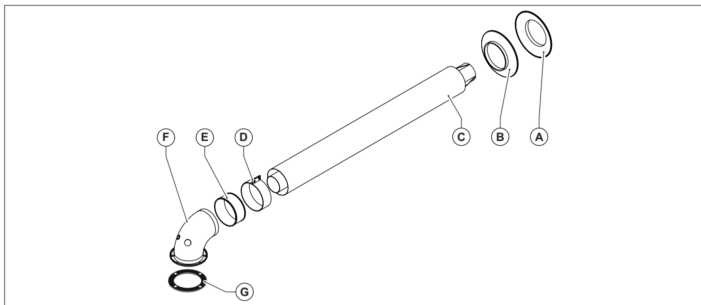
Рис. 10 Коаксильный комплект 6KITCON00A
