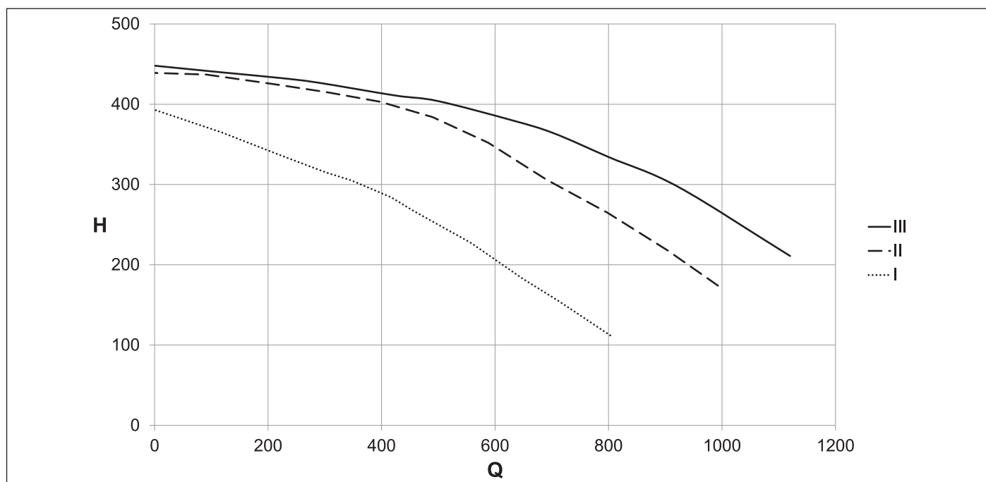
Рис. 19 Располагаемый напор CTFS 32
